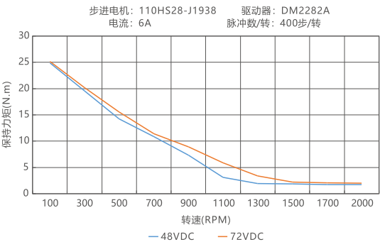
力矩曲线图
