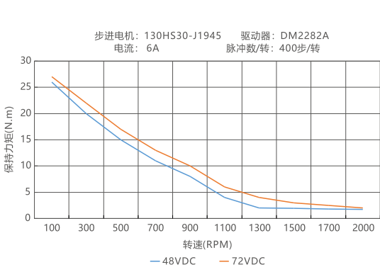
力矩曲线图
