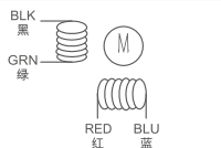
接线图
