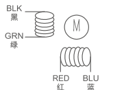
接线图
