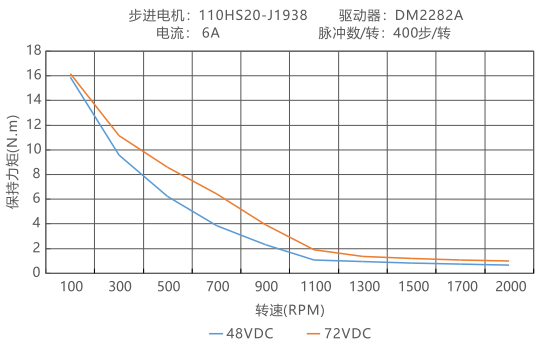
力矩曲线图
